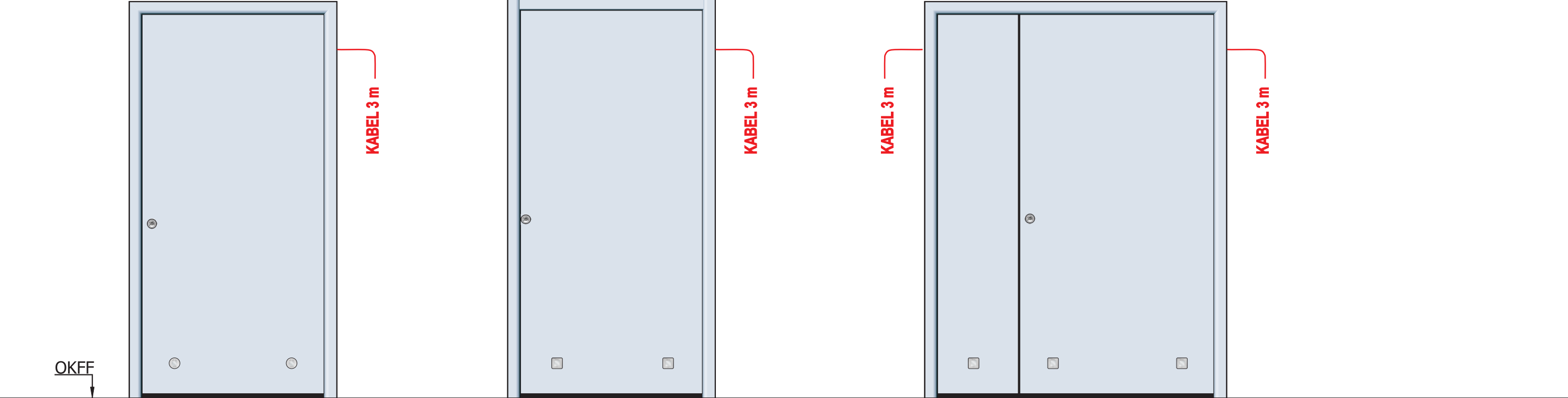
Einflügelige Tür
