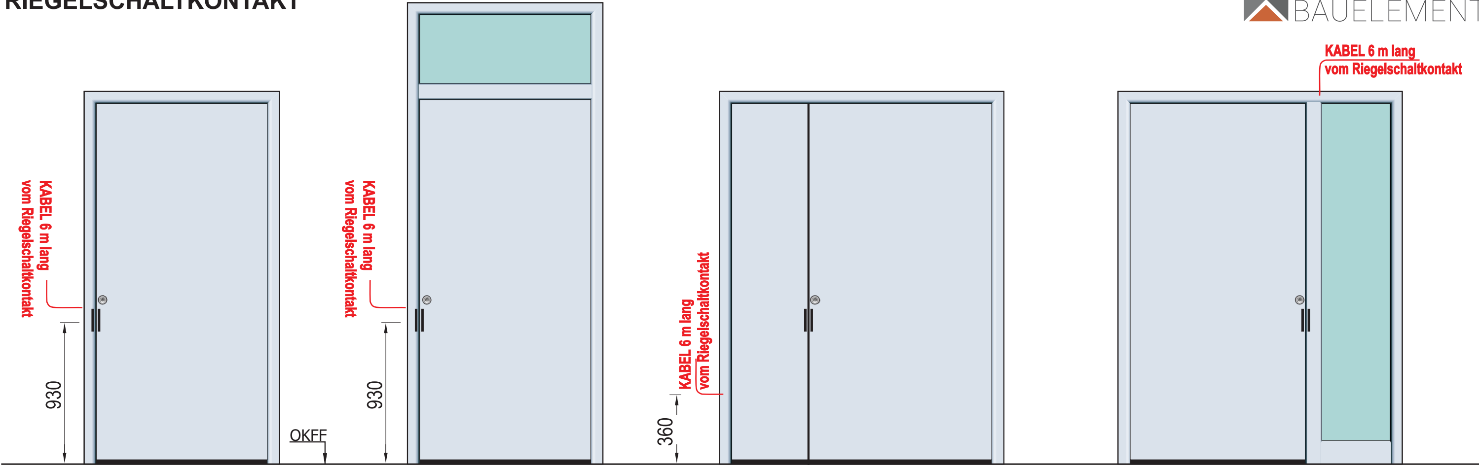
Einflügelige Tür mit eine Seitenteil
